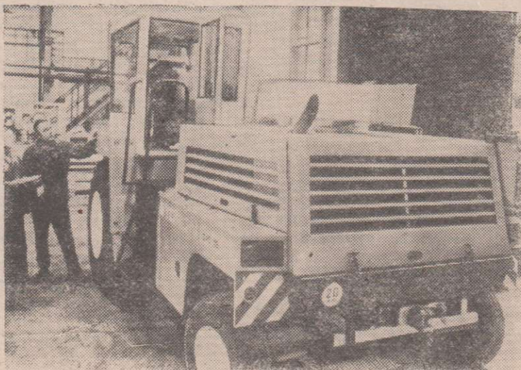
ЧССР. На заводе «Агрострой» в Простеевце начал выпуск нового силосоуборочного комбайна «СПС-35», созданного специалистами Венгрии, Польши и Советского Союза. Машина выгодно отличается от своих предшественниц: она на 600 килограммов легче и потребляет на 15 процентов меньше горючего при движении, мощность которого увеличена почти на треть. «СПС-35» будет поставляться в страны-члены СЭВ. На снимке: идет сборка комбайна «СПС-35».
